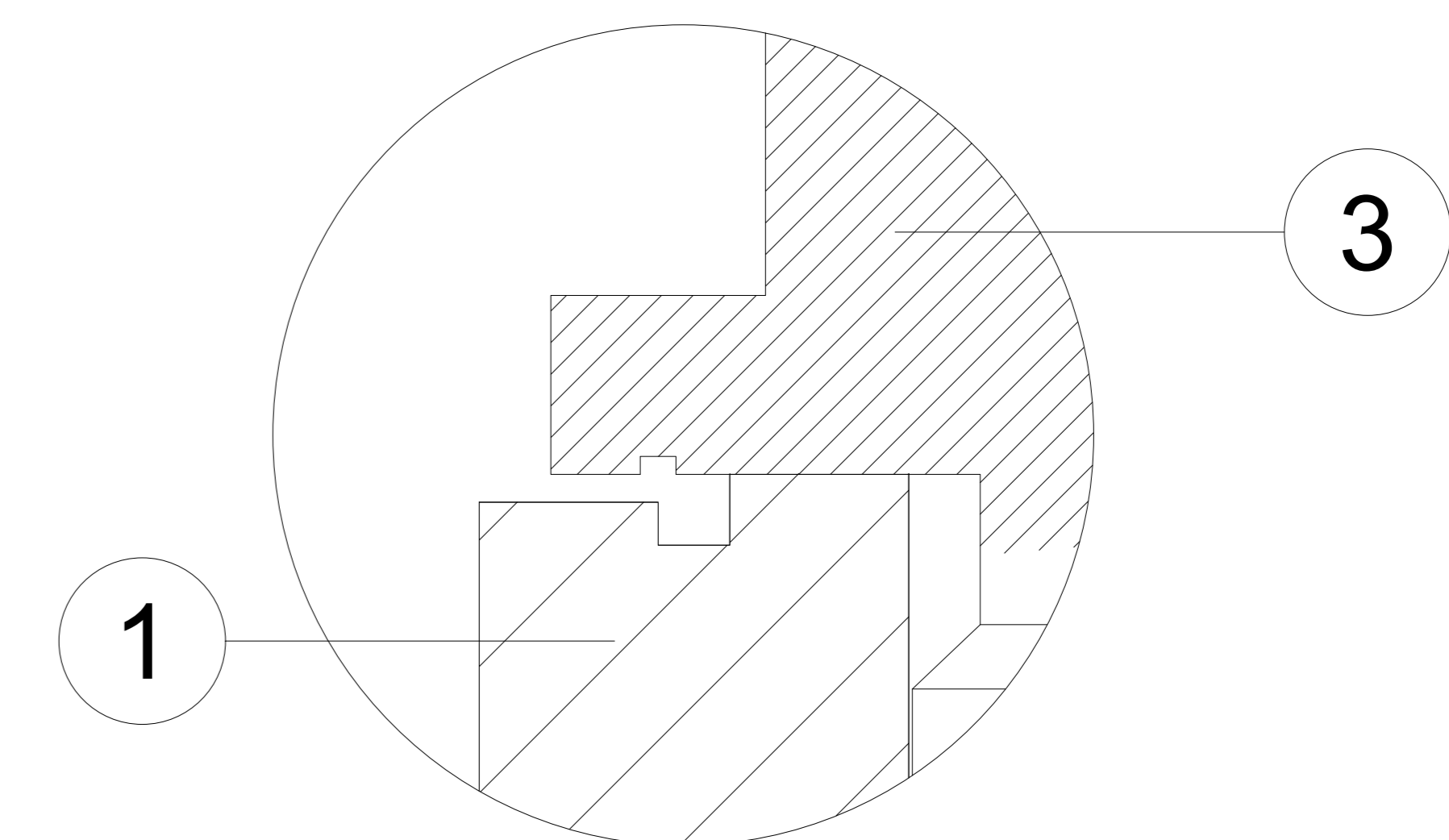
DETALLE -A- (SELLO)
