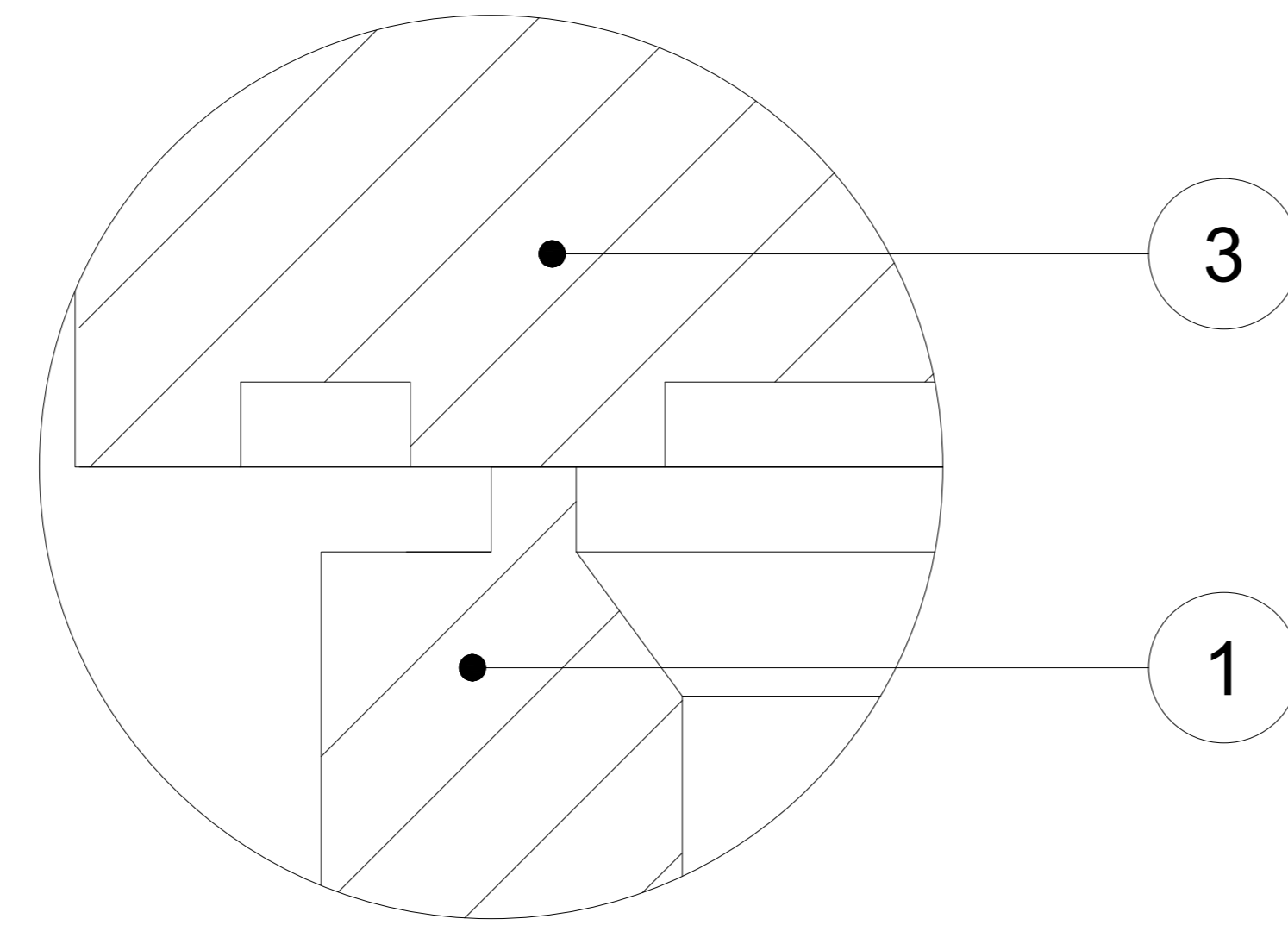
DETALLE -A- (SELLO)
