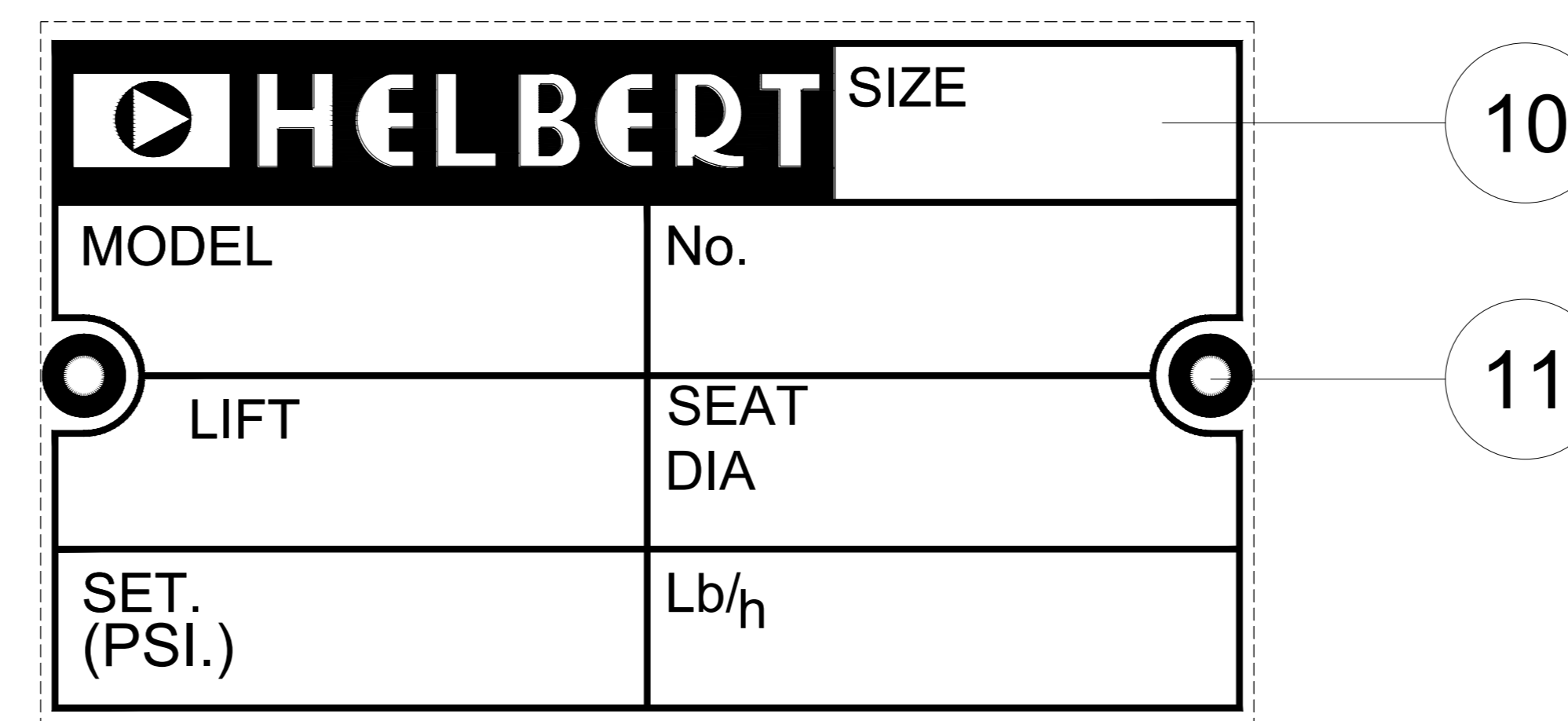
DETALLE -B- (PLACA DE IDENTIFICACIÓN)
