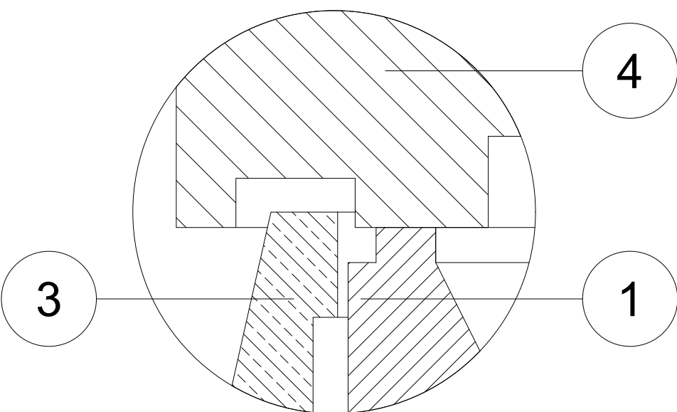
DETALLE -A- (SELLO)
